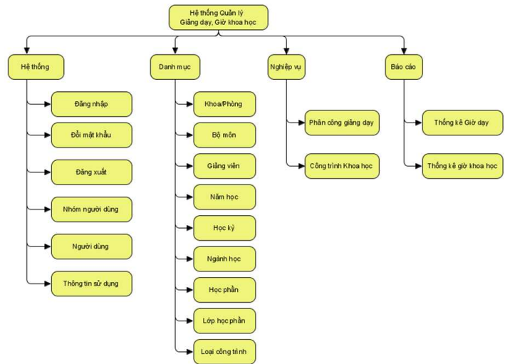
Hình 1. Sơ đồ phân rã chức năng của phần mềm
